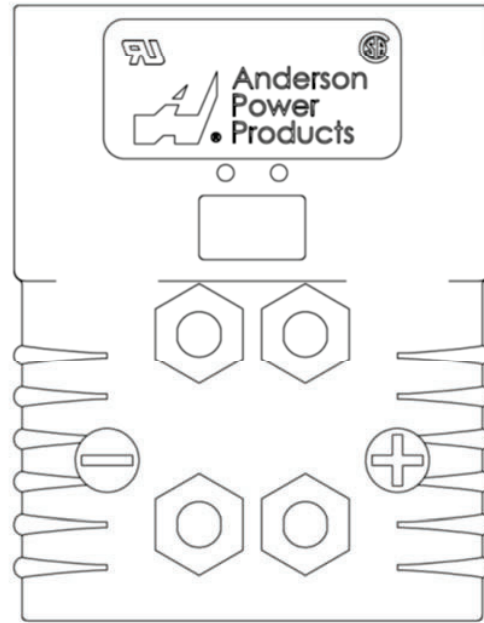
SBE®160 - SBX®175
