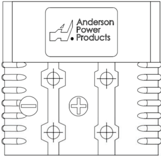
SB®175 - 3 Pole
