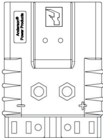
SBE®60 - SBO®80
