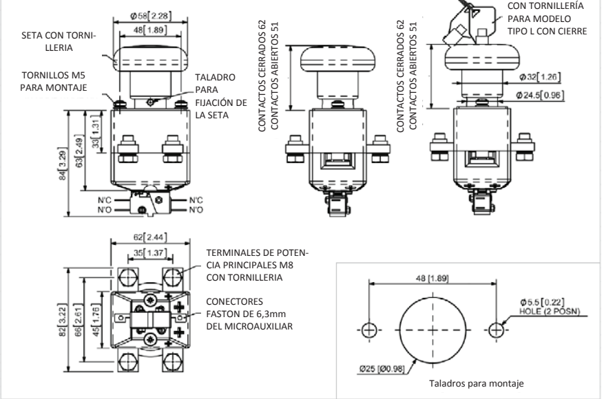
Dimensiones en mm [inches]
